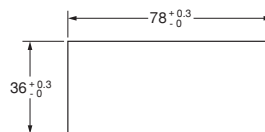
取り付け穴加工寸法
